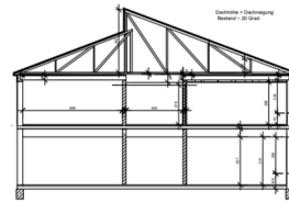
Querschnitt Bestand
