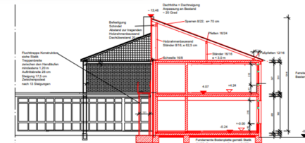
Querschnitt Erweiterung
